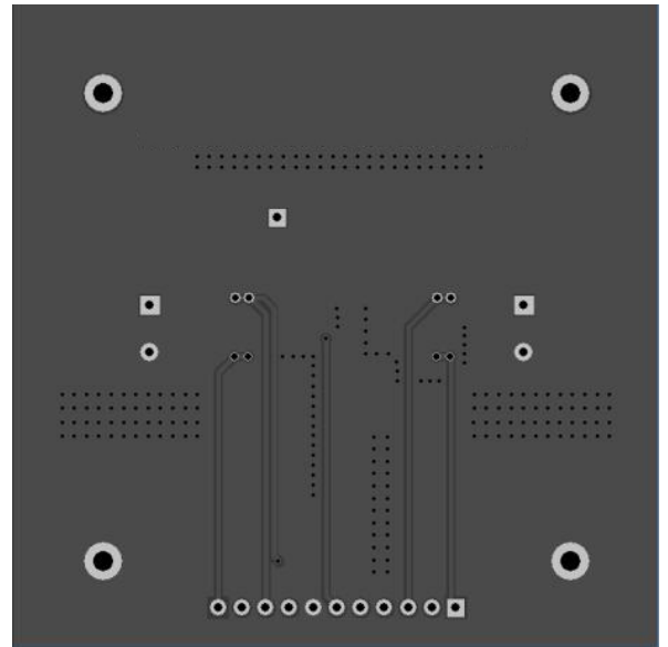
Bottom Layer
